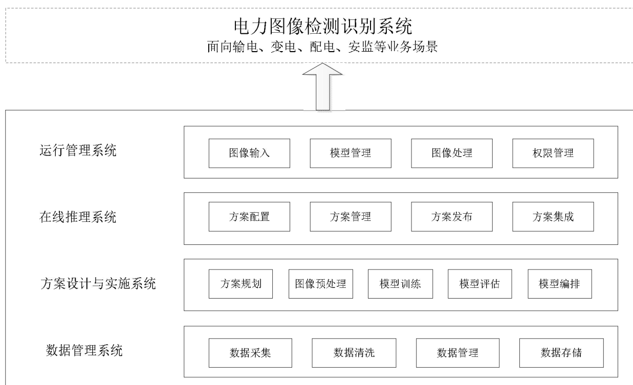
图 1 电力图像检测识别系统架构
